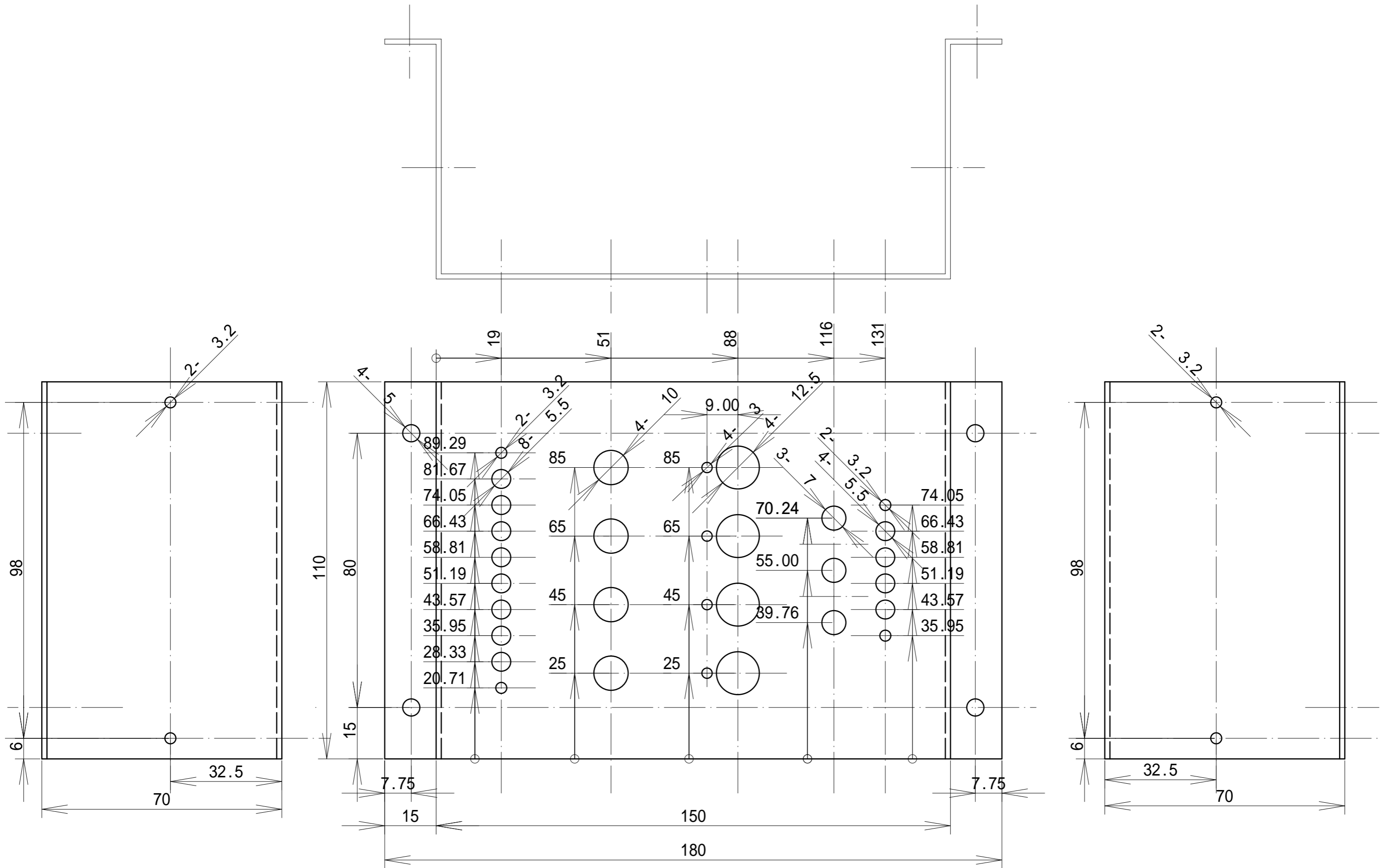
正面図
