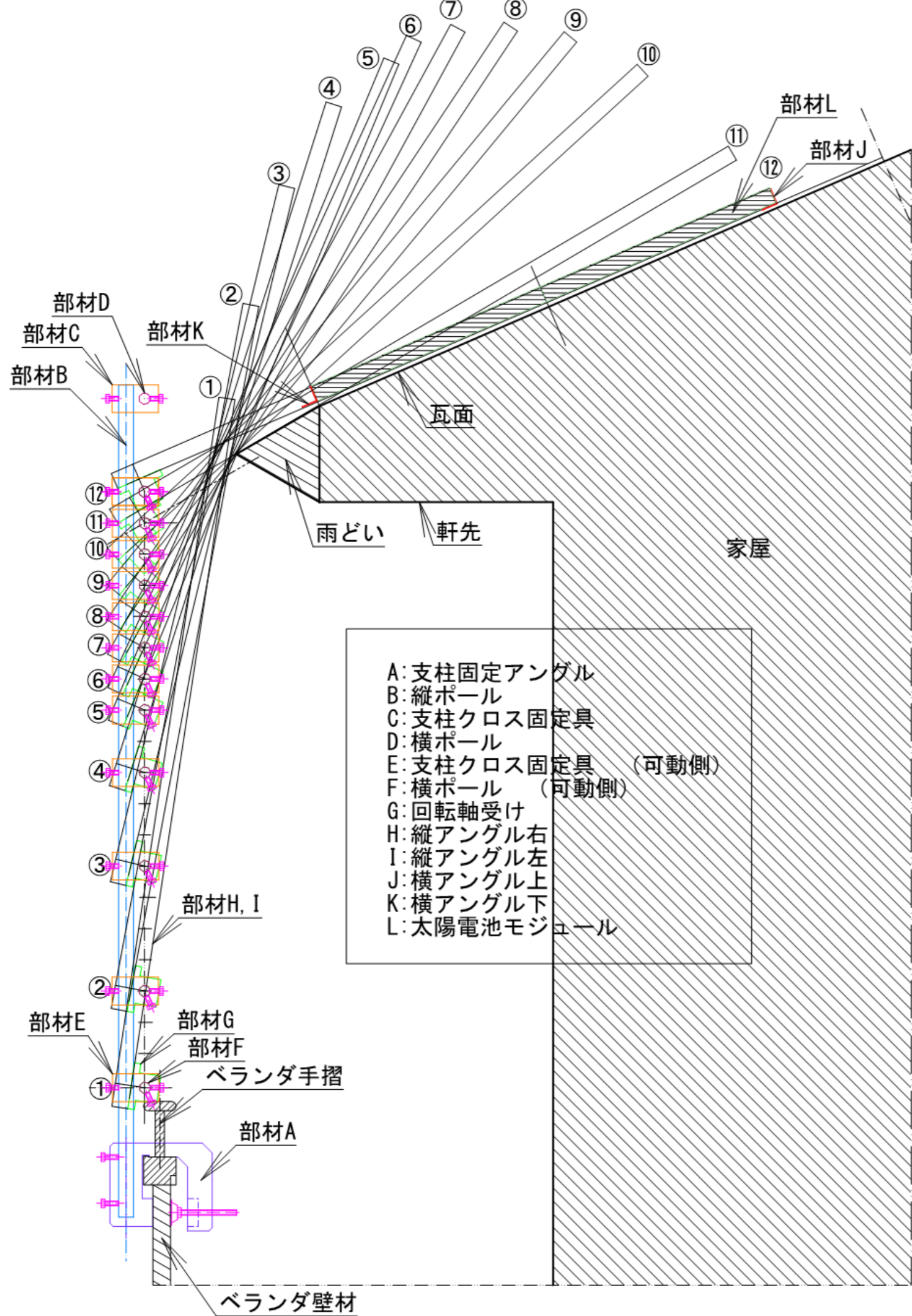
組立図 & 動作説明図
